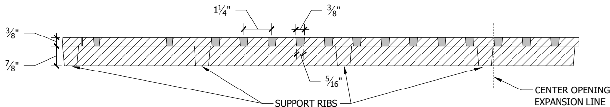
Section A-A'
