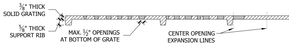
Section A-A'
