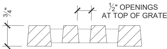
Cross Section Scale: 6" = 1' 0"
