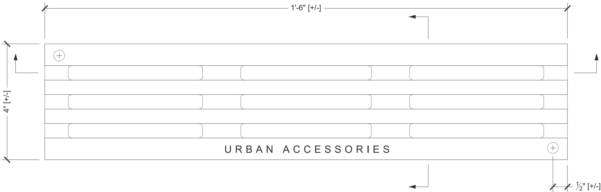
Plan Scale: 6" = 1' 0"
