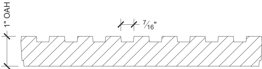
Cross Section Scale: 6" = 1' 0"
