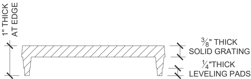
Cross Section Scale: 6" = 1' 0"
