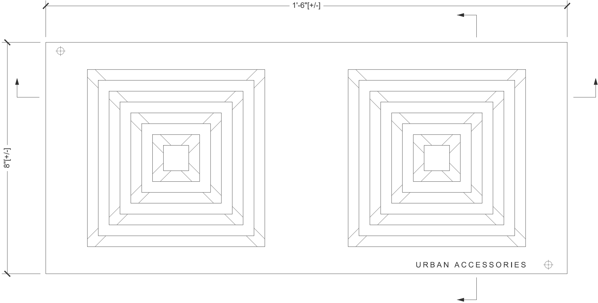
Plan Scale: 6" = 1' 0"
