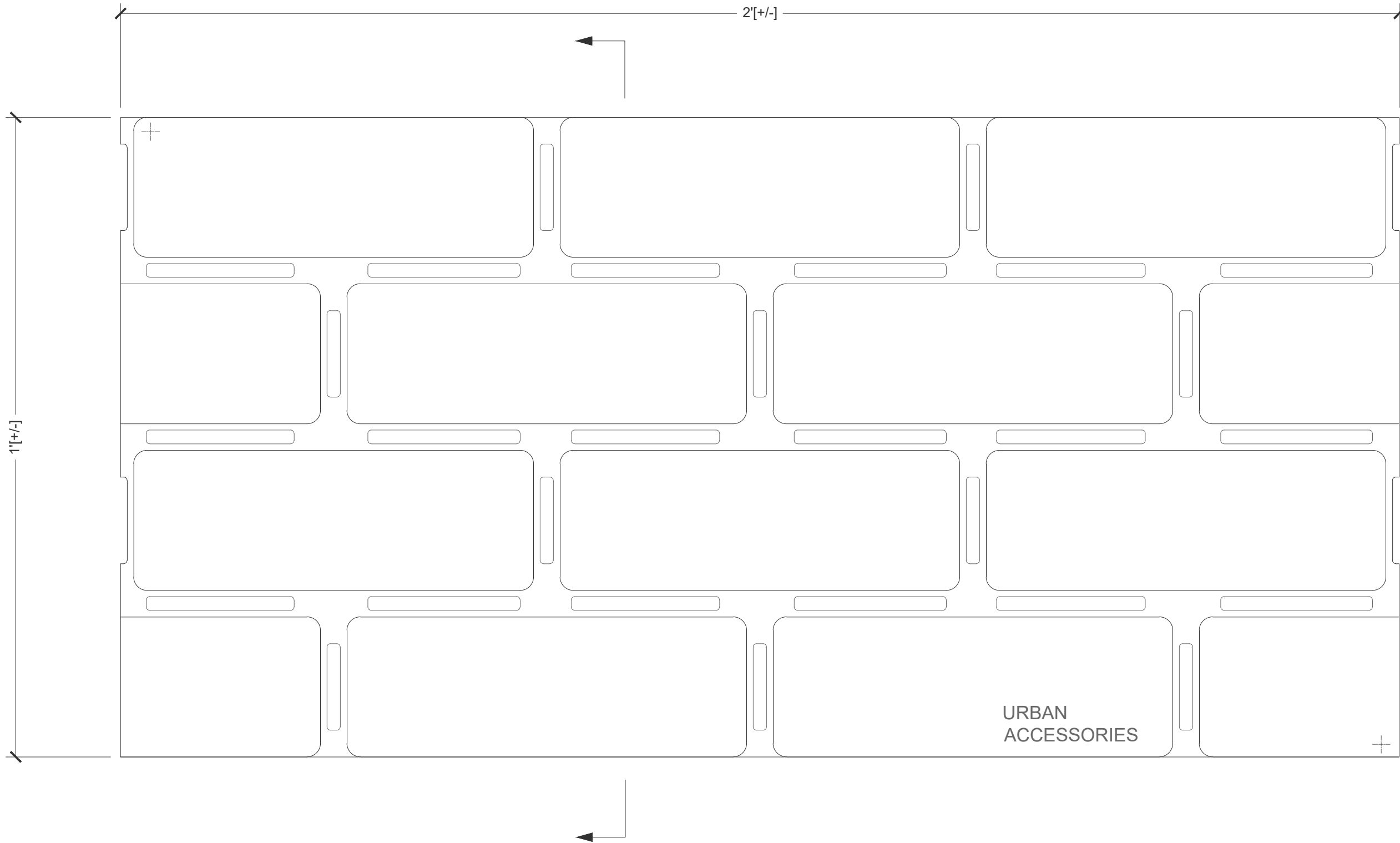
Plan Scale: 6" = 1' 0"
