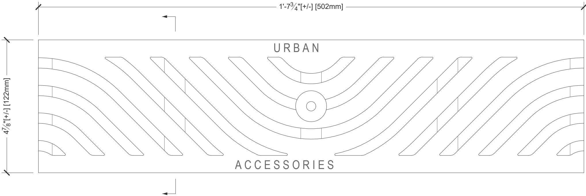
Plan Scale: 6" = 1' 0"
