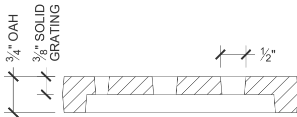
Cross Section Scale: 6" = 1' 0"
