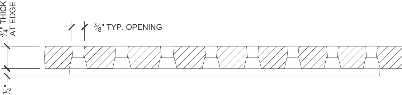
Cross Section Scale: 6" = 1' 0"
