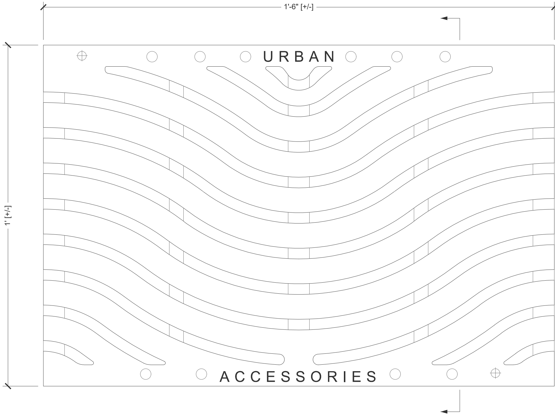
Plan Scale: 6" = 1' 0"
