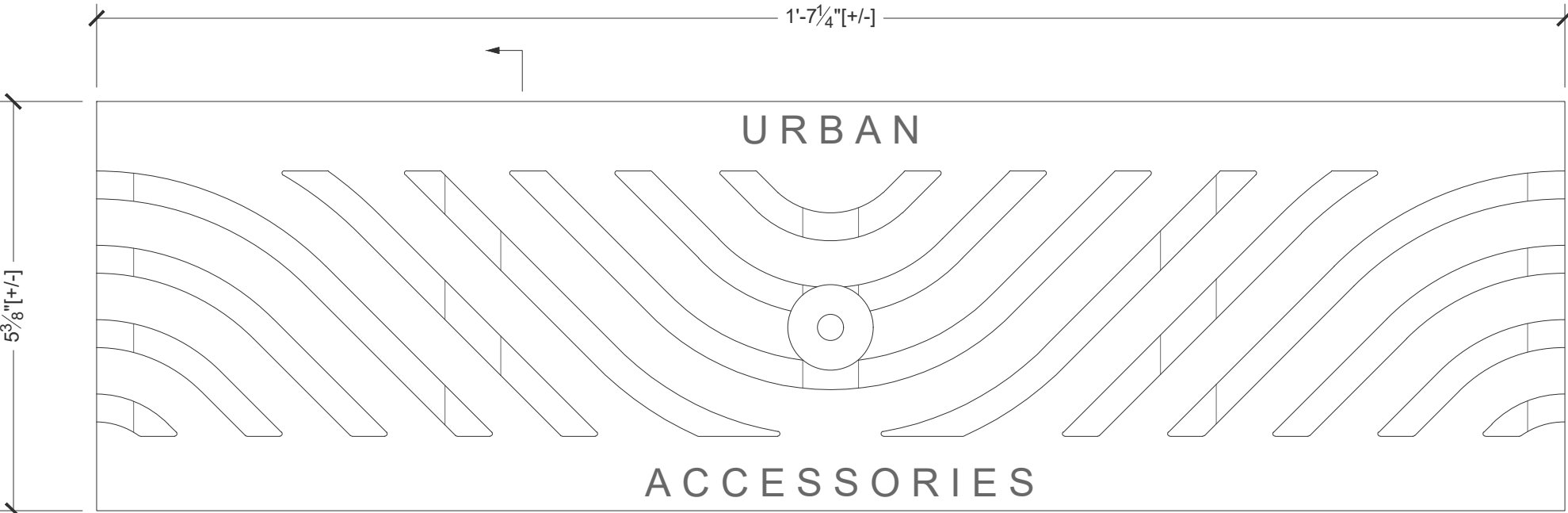
Plan Scale: 6" = 1' 0"
