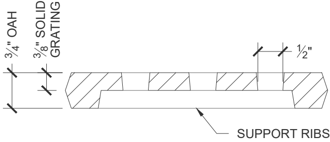
Cross Section Scale: 6" = 1' 0"
